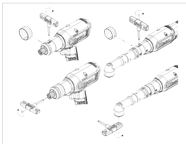
Abb. 2-3: Drehmoment einstellen
