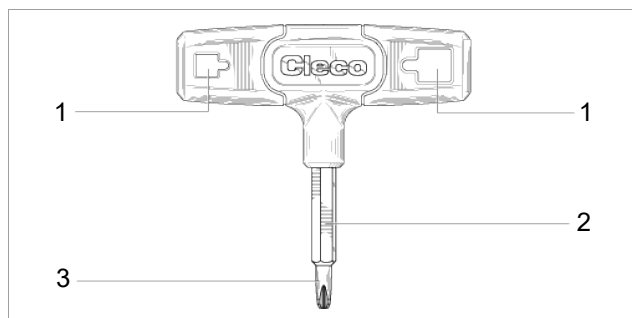
Abb. 5-2: 调整工具 订购号 T50-1001619
