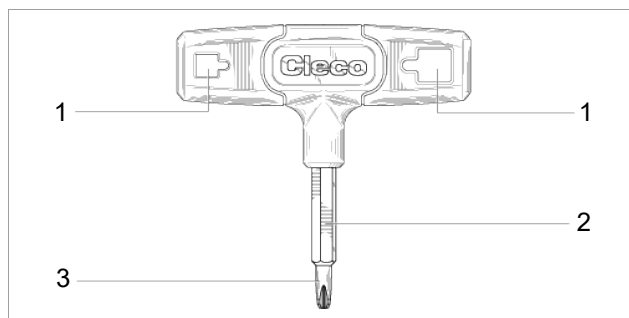
Abb. 2-2: Einstellwerkzeug Bestell-Nr. T50-1001619
