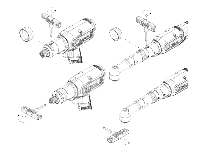
插图 5-3: 设置扭矩
