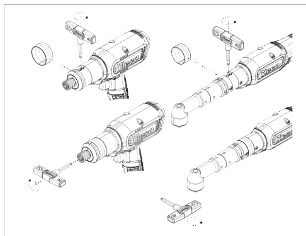
Fig. 3-3: ajuste del torque
