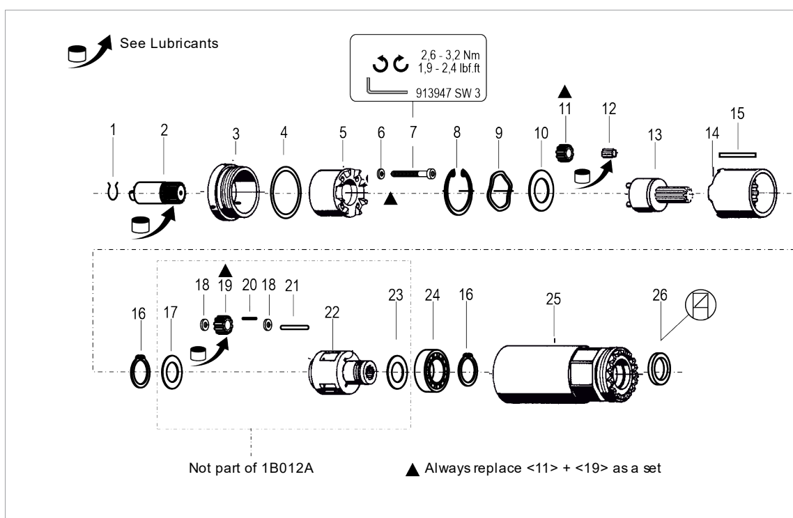
Fig. 2-1: Assembly 1B(...)A
