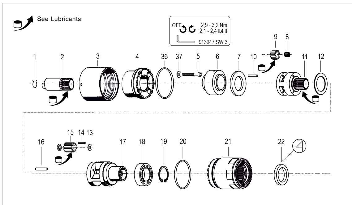
Fig. 3-1: Assembly 2B110A
