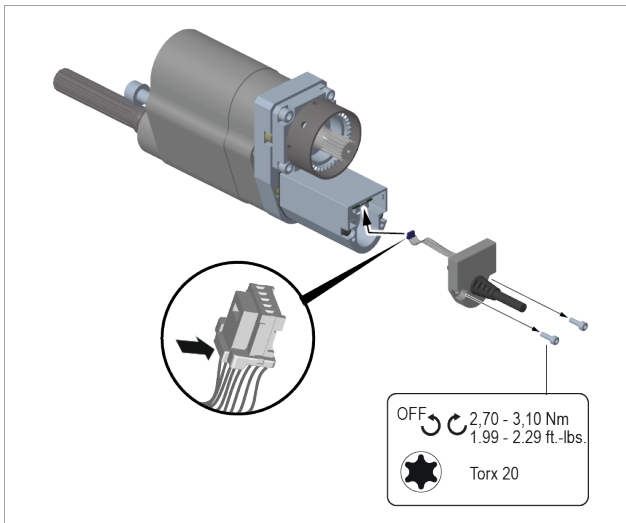
Fig. 8-1: Substituir o cabo
