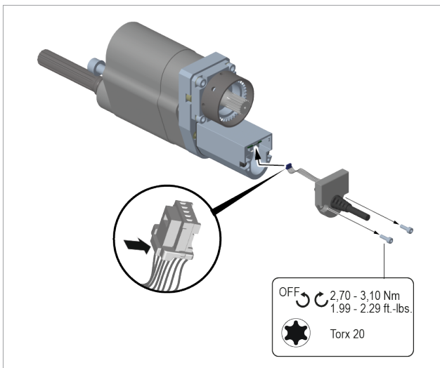
Fig. 5-1: Sostituzione del cavo
