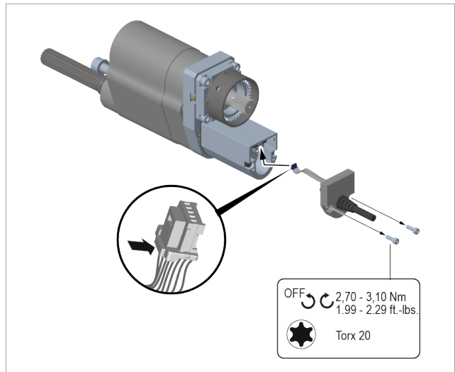
Abb. 2-1: Kabel tauschen
