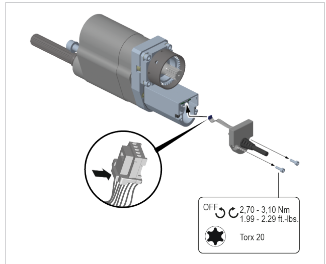
插图 6-1: 更换电缆
