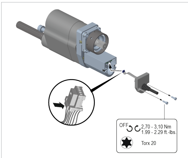
Fig. 4-1 : Remplacer le câble
