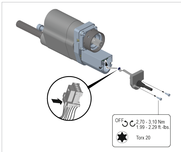
Rys. 7-1: Wymienić kabel
