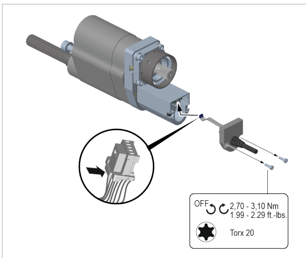
Fig. 3-1: Cambiar el cable
