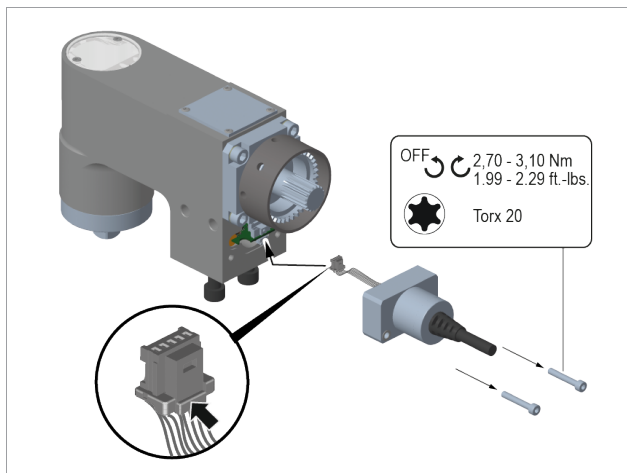
Rys. 7-1: Wymienić kabel
