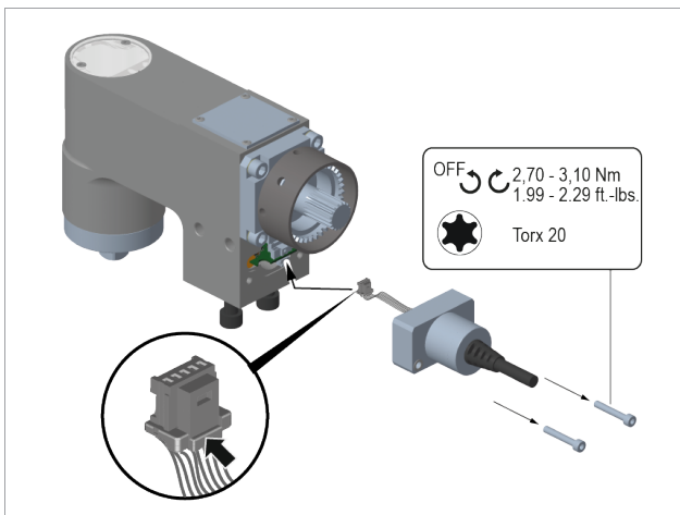
Fig. 4-1 : Remplacer le câble
