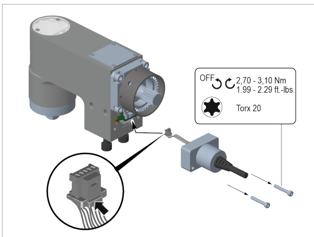
Fig. 5-1: Sostituzione del cavo
