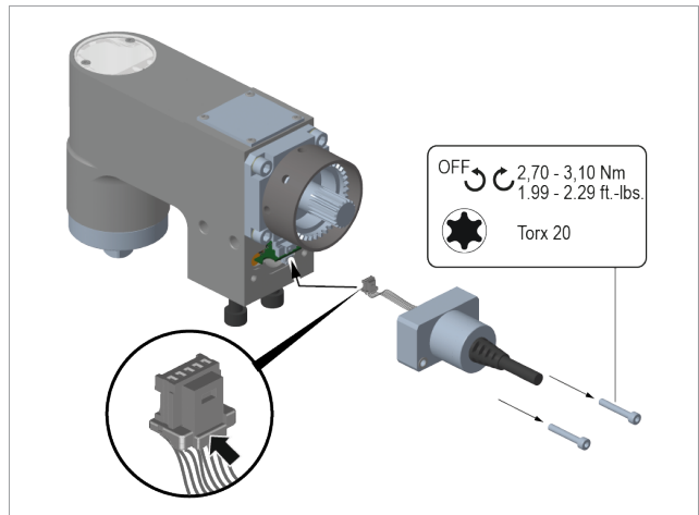
Abb. 2-1: Kabel tauschen
