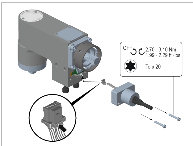
Fig. 3-1: Cambiar el cable
