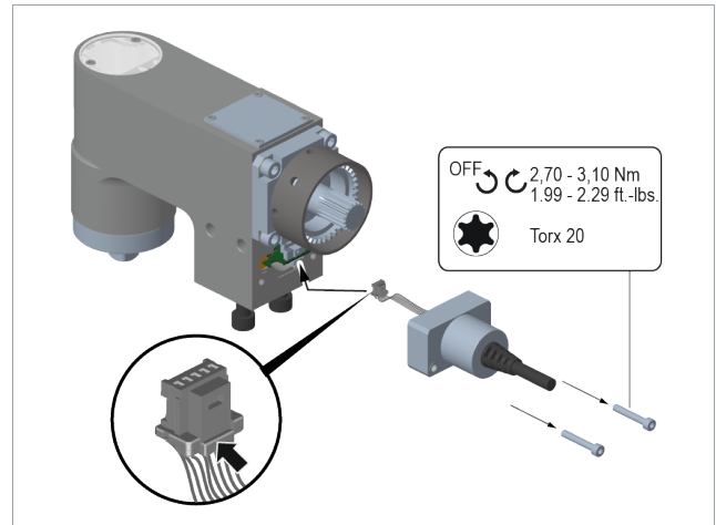
插图 6-1: 更换电缆
