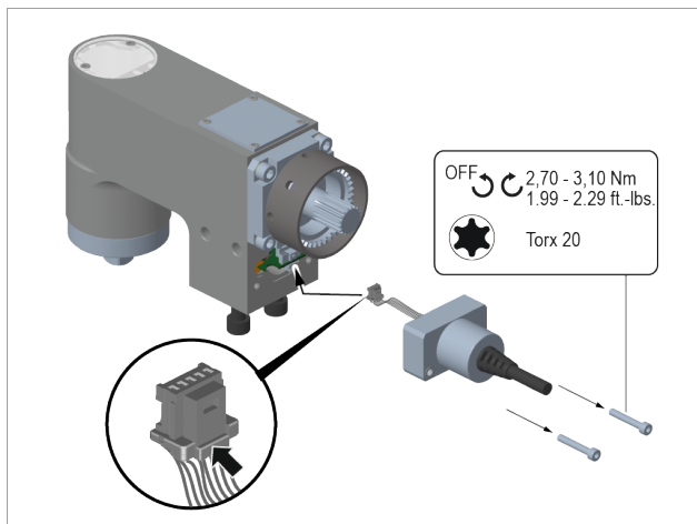
9-1. ábra: Vezeték cseréje
