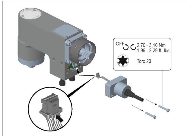
Fig. 8-1: Substituir o cabo
