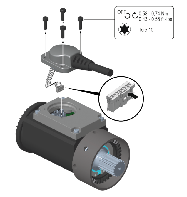
Abb. 2-1: Kabel tauschen
